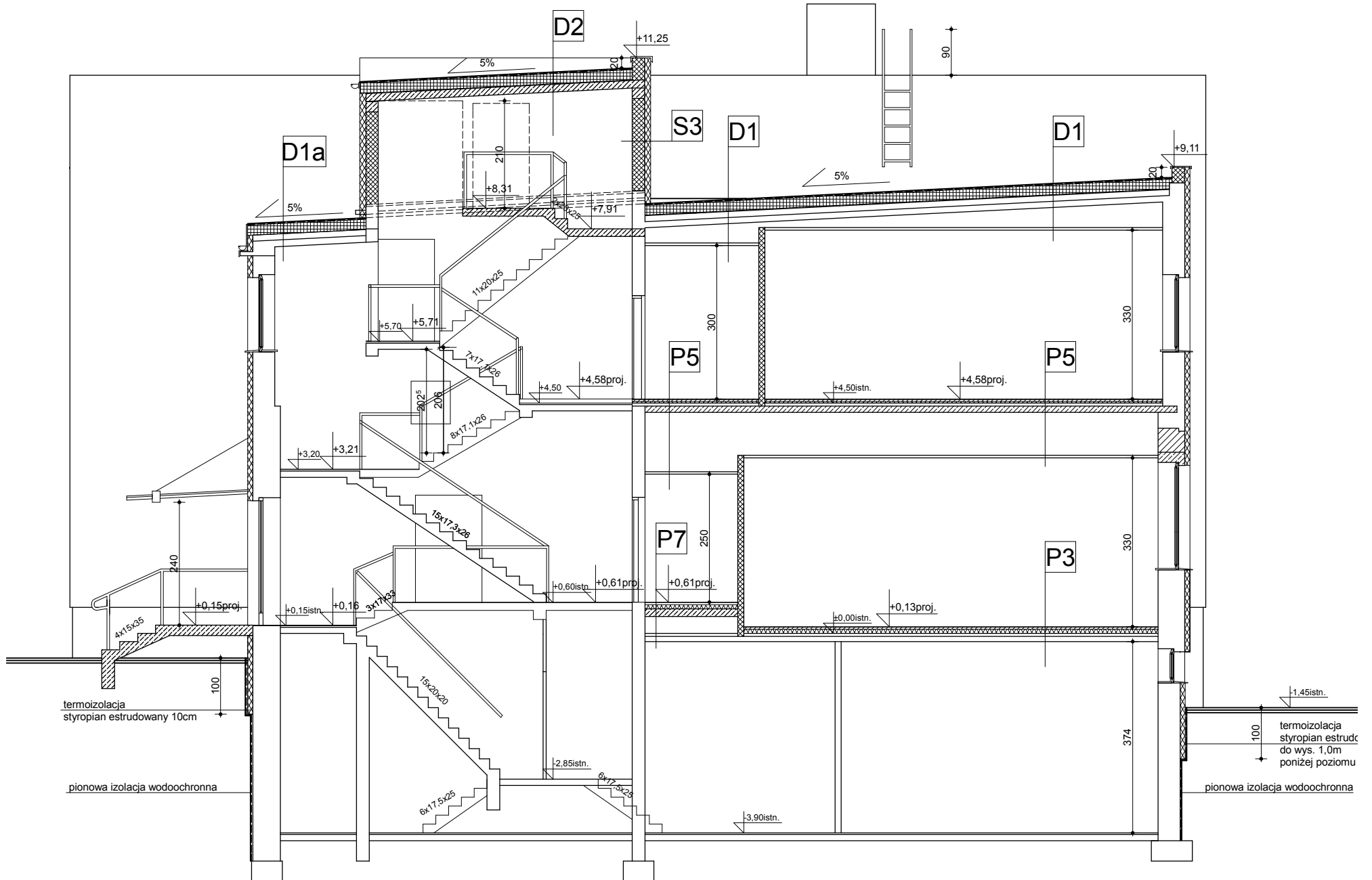
Przekrój C - C 1:100
